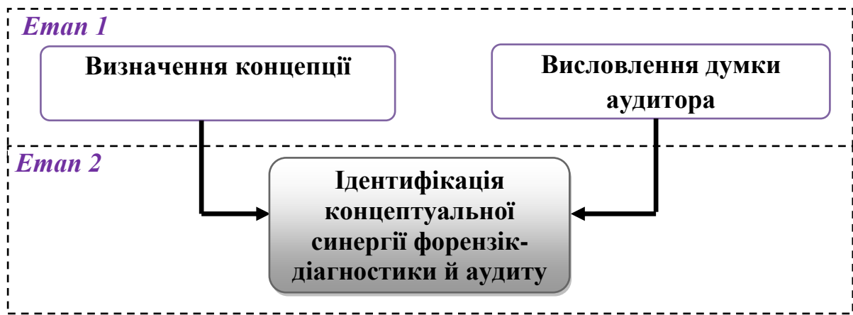
Рис. 3. Логіка визначення концептуальної моделі синергії форензик-діагностики та аудиту
