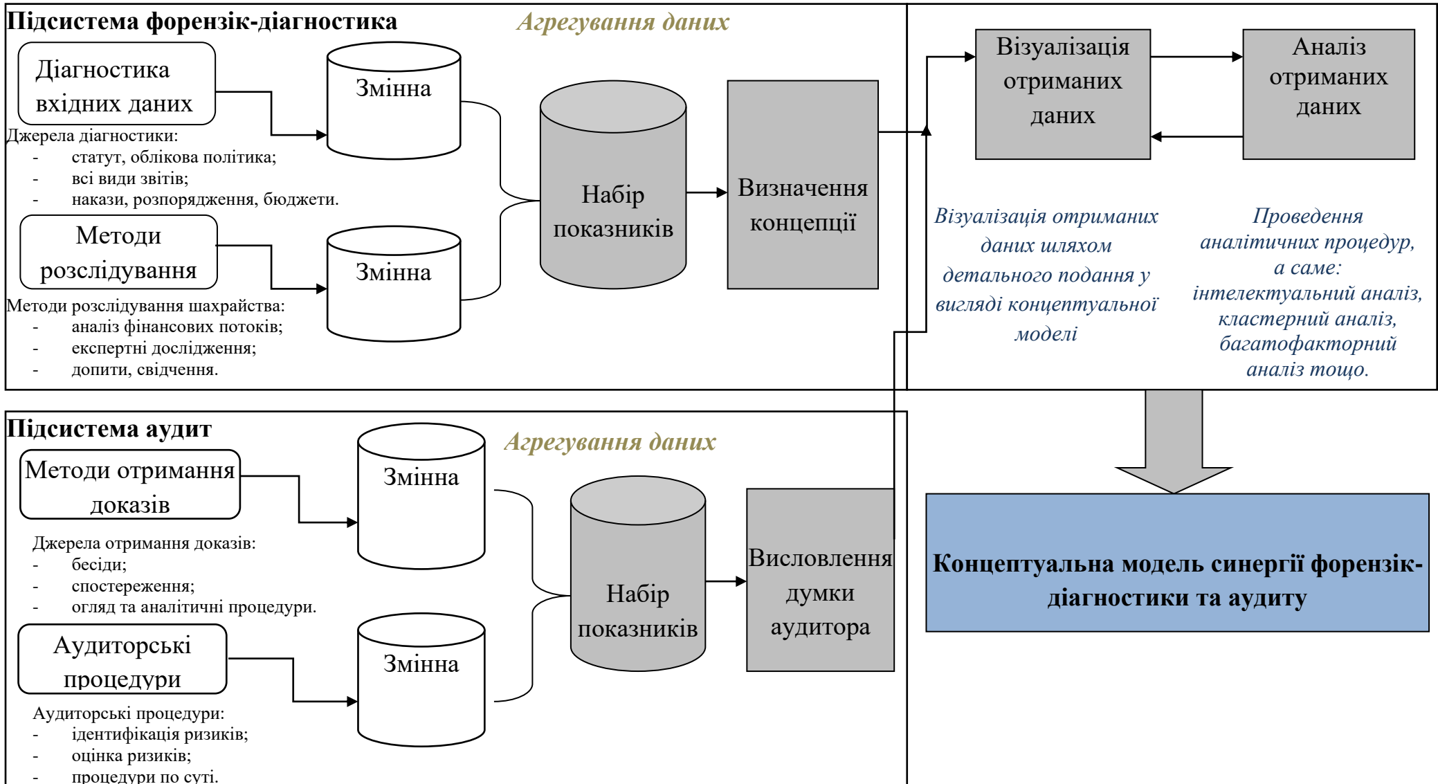
Рис. 2. Механізм побудови концептуальної моделі синергії форензик-діагностики та аудиту Джерело: Розроблено автором.
