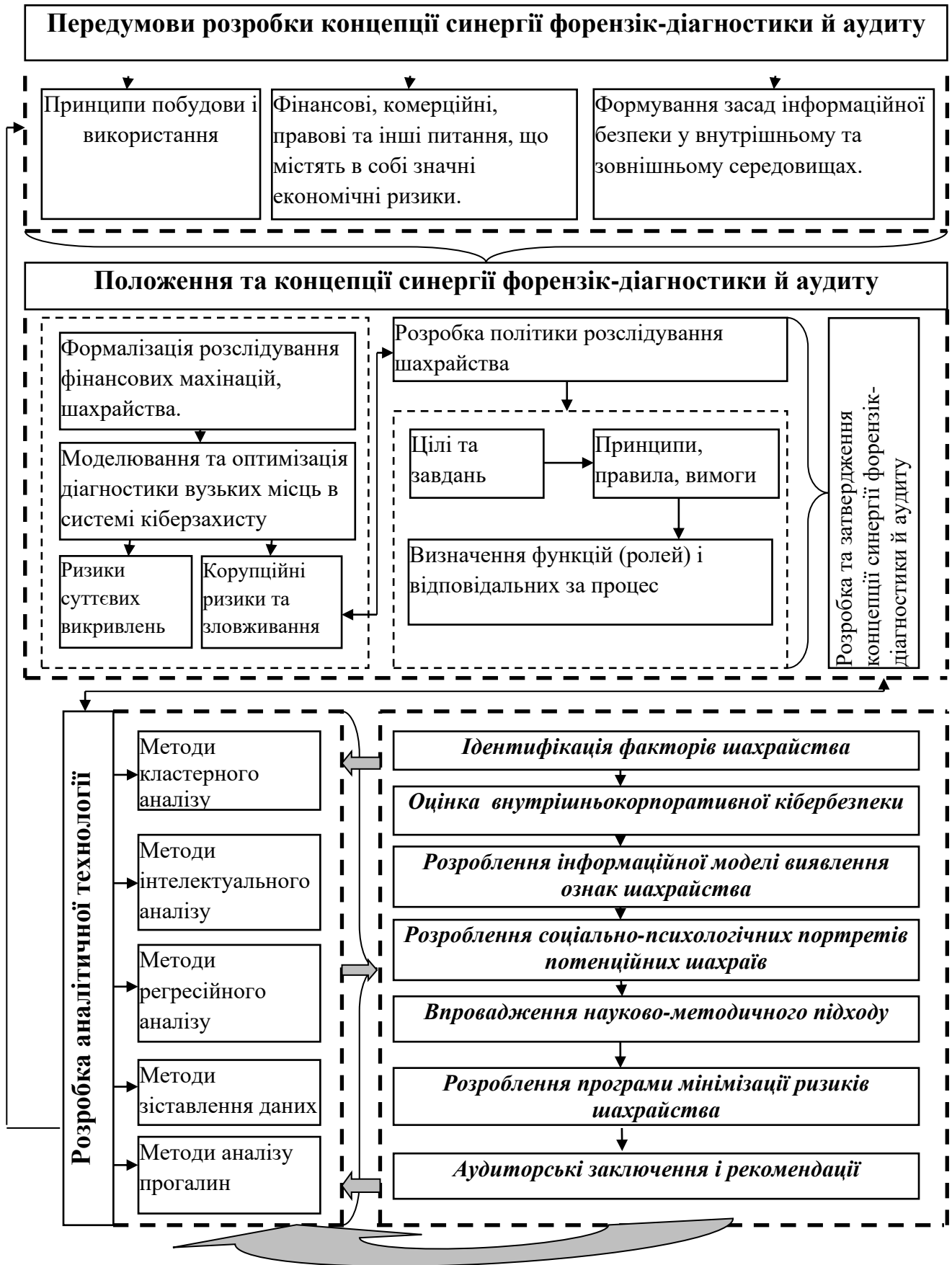
Рис. 4. Концептуальна модель синергії форензик-діагностики та аудиту
